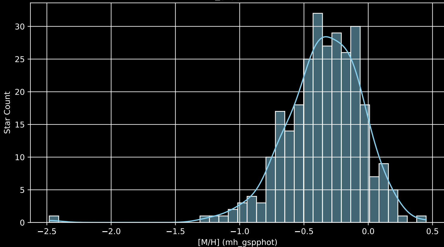
GALAH DR4 Field: [410] [M/H] (mh_gspphot) (n= 285)
