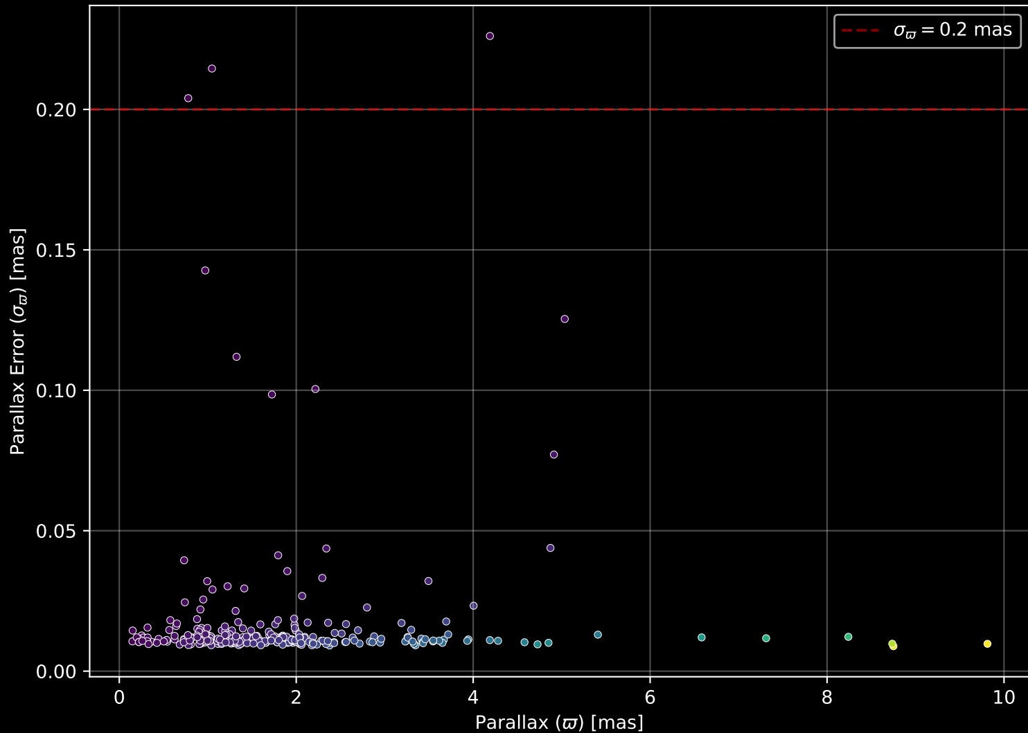
GALAH DR4 Field: [410] Parallax Quality (n= 287)
