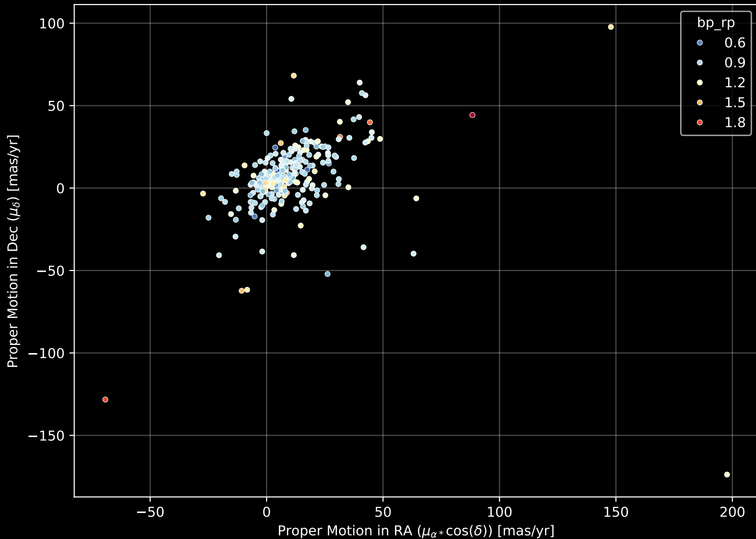
GALAH DR4 Field: [410] Proper Motion Diagram (n= 287)
