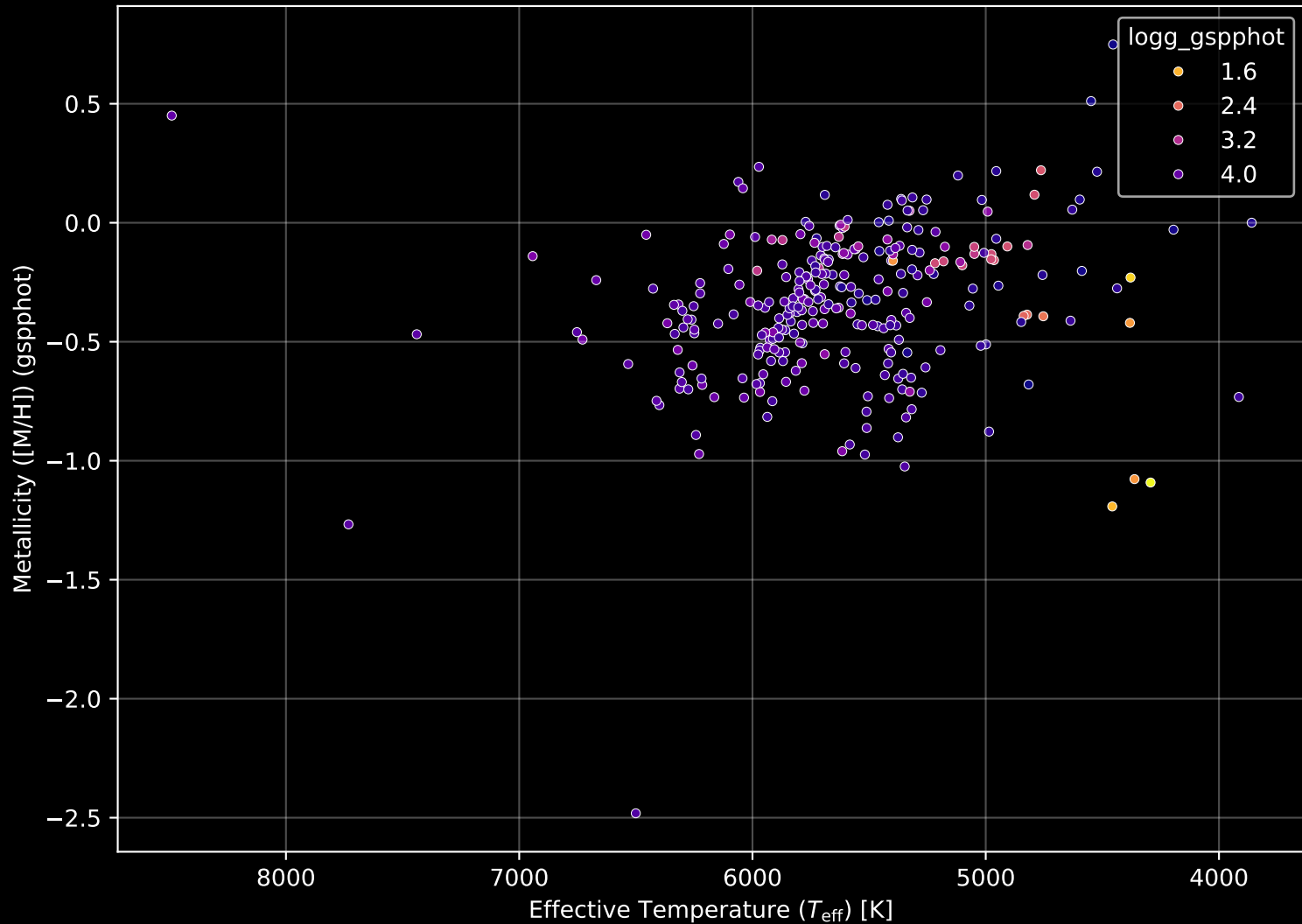
GALAH DR4 Field: [410] Stellar Population Parameters (n= 287)
